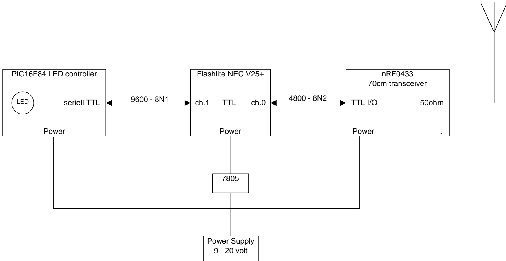
Blokkskjema over Flashlite- delen av LED kontroll systemet.
